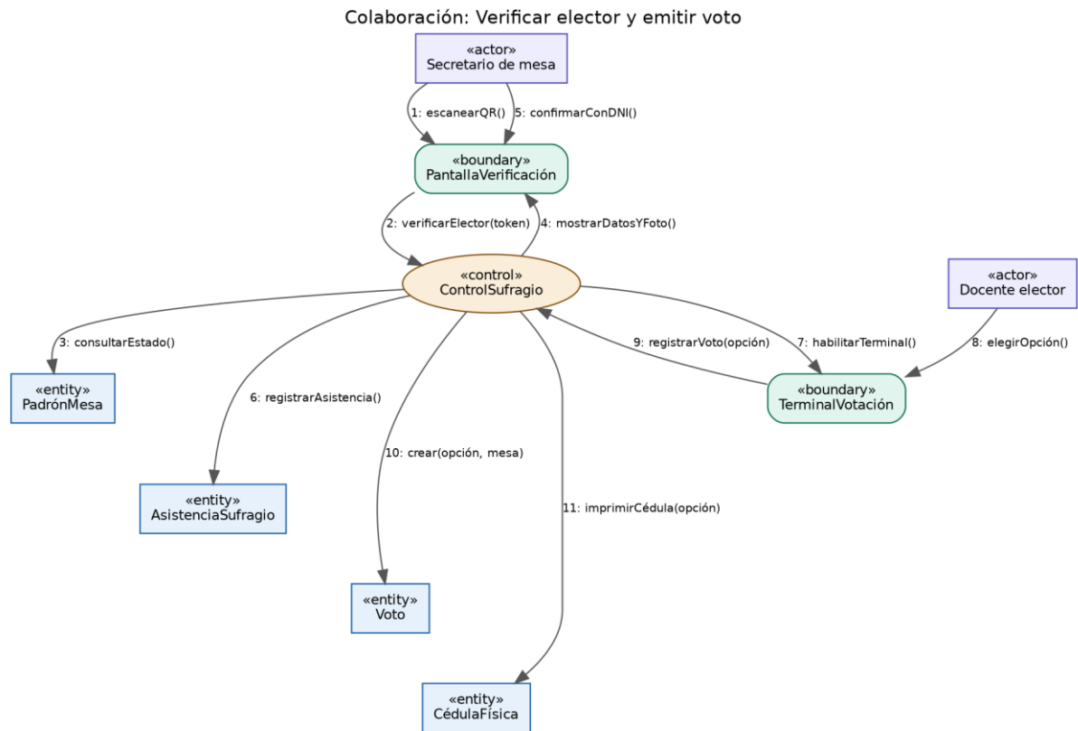
Figura 7. Diagrama de colaboración de CUS09 y CUS10.
