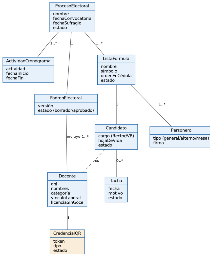
Figura 2. Modelo de dominio (1 de 2): proceso, padrón e inscripción. En color, las clases que propone el sistema.
