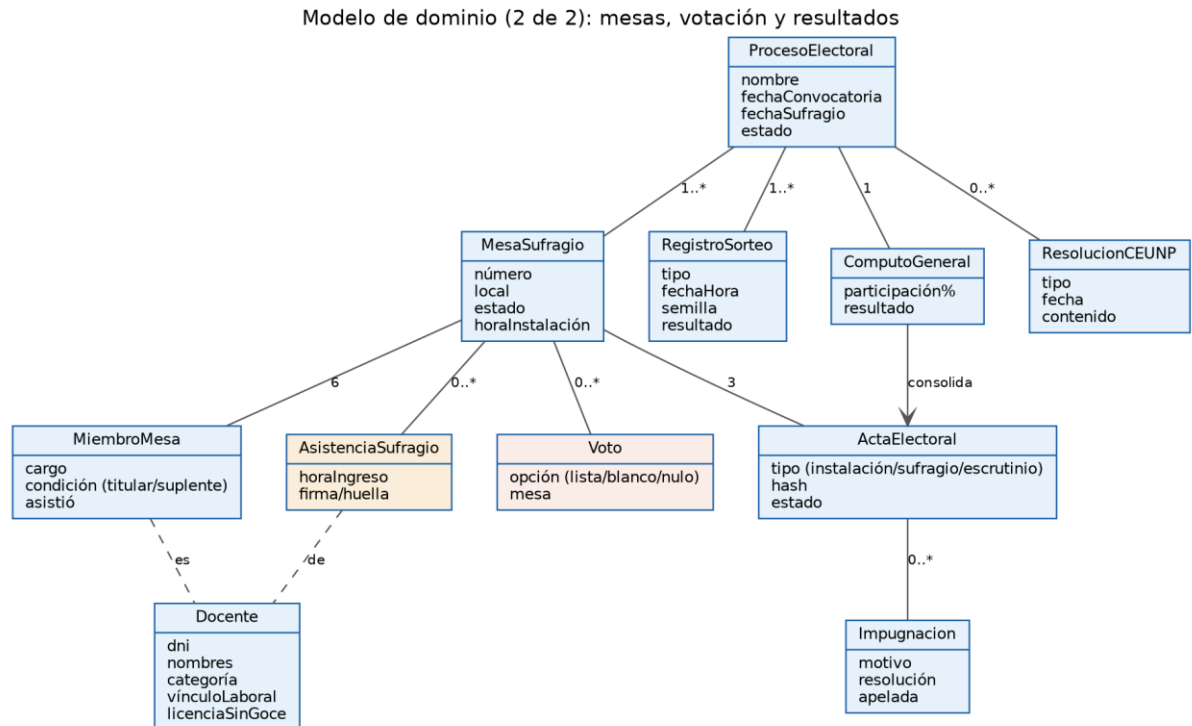
Figura 3. Modelo de dominio (2 de 2): mesas, votación y resultados. La clase Voto no tiene ninguna relación con Docente ni con AsistenciaSufragio, para preservar el secreto del voto.
