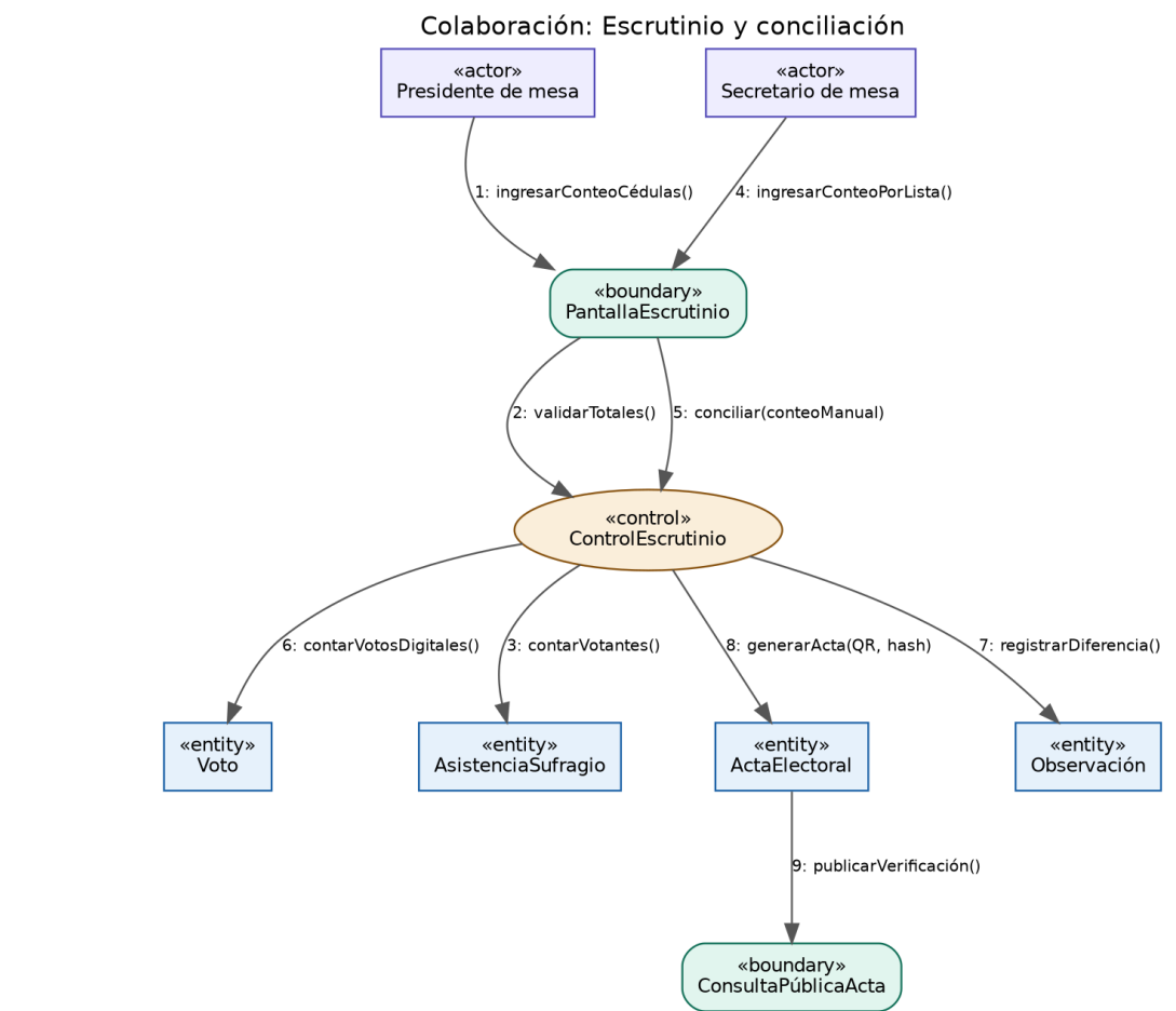
Figura 8. Diagrama de colaboración de CUS12.
