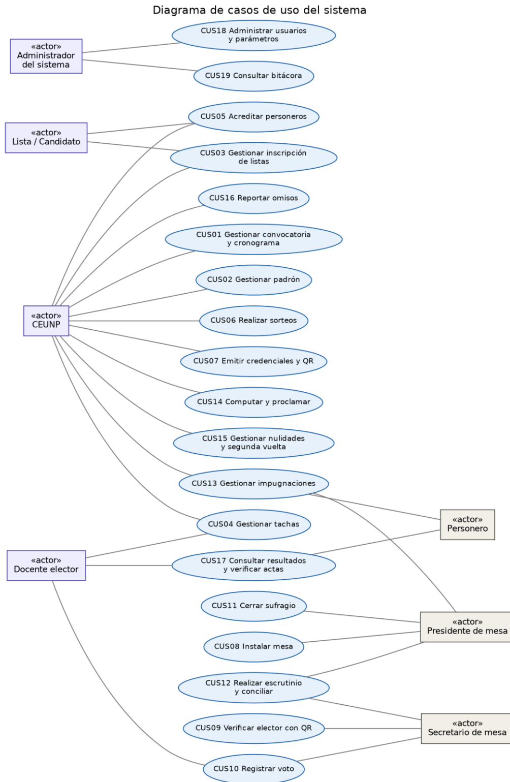
Figura 6. Diagrama de casos de uso del sistema.
