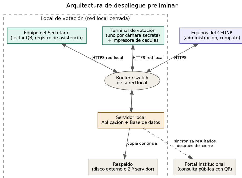
Figura 9. Arquitectura de despliegue preliminar.
